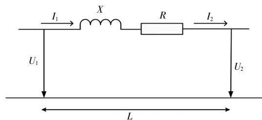
图 1 一字型单相线路传输模型
