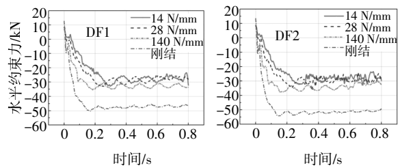
(b) DF1 和 DF2 试件不同水平约束刚度
