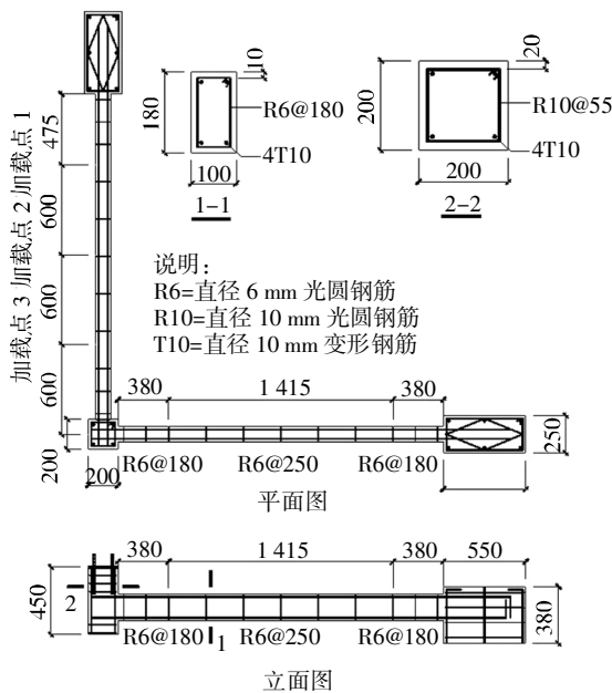
图 3 DF1 试件配筋示意图(单位:mm) Fig.3 Dimensions and cross sectional details of DF1 (Unit: mm)
