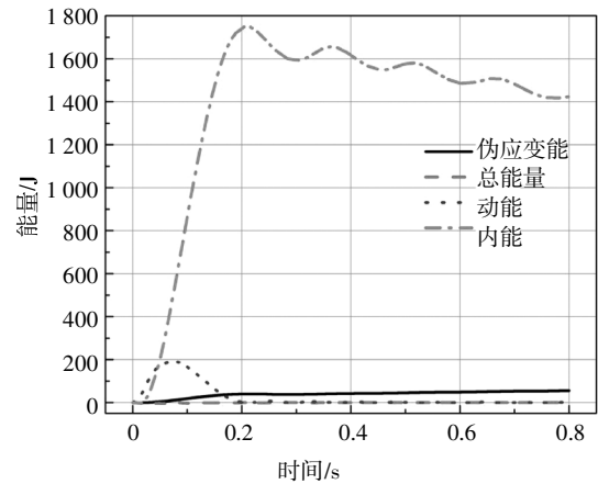
图7 DF1 模型的历史能量曲线
