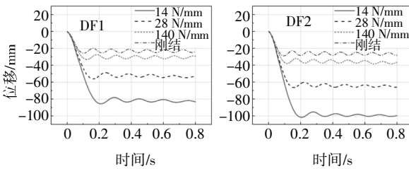
(b) DF1 和 DF2 试件不同水平约束刚度
