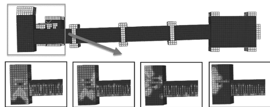
失效时长<math><0.17T</math> 失效时长 0.57T 失效时长 1.07T 失效时长 2.07T
