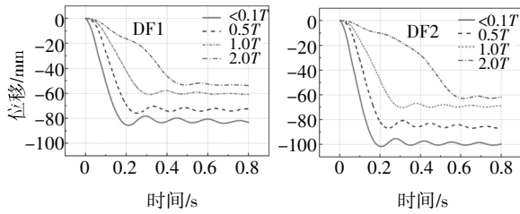
(a) DF1 和 DF2 试件不同失效时间
