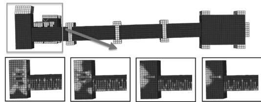
失效时长<math><0.17T</math> 失效时长 0.57T 失效时长 1.07T 失效时长 2.07T
