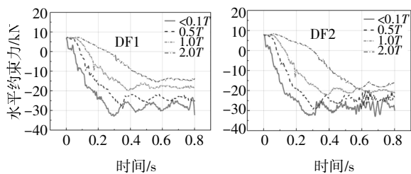
(a) DF1 和 DF2 试件不同失效时间
