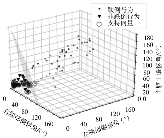
图 9 训练样本集二分类效果
