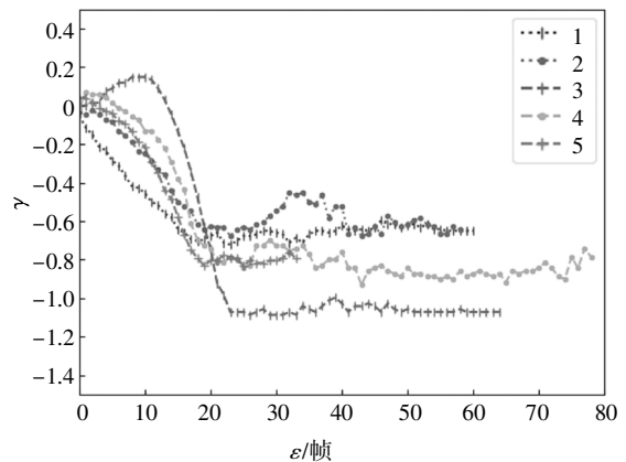
图 11 \gamma - \varepsilon 关系图
