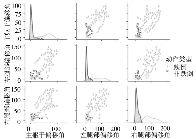
图 8 人体倾斜姿态特征向量多属性关系图(单位:°)
